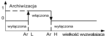
Rys. 29. Typy archiwizacji: a) n_on b) noFF c) on d) Off
