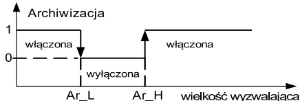
Rys. 29. Typy archiwizacji: a) n_on b) noFF c) on d) Off
