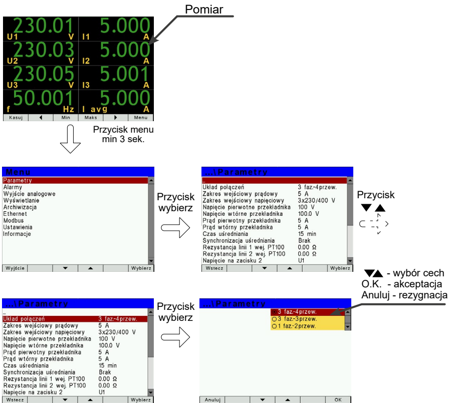
Rys. 23. Ekran trybu Parametry
