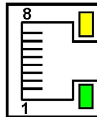
Rys. 46. Widok i numeracja pinów gniazda RJ45 miernika
